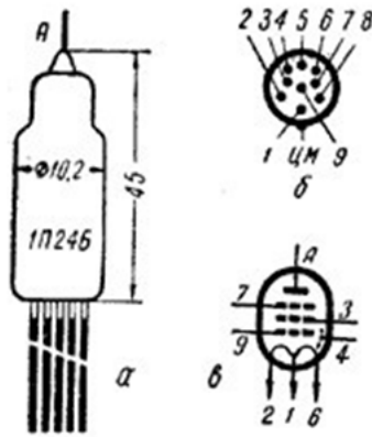
Рис. 78. Лампа 1П24Б:
